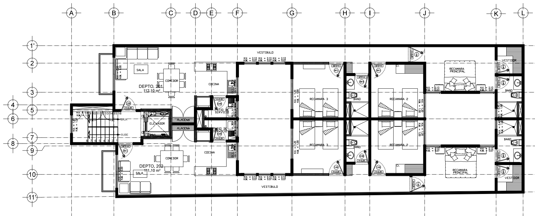
PLANTA TIPO MÓNACO 300
