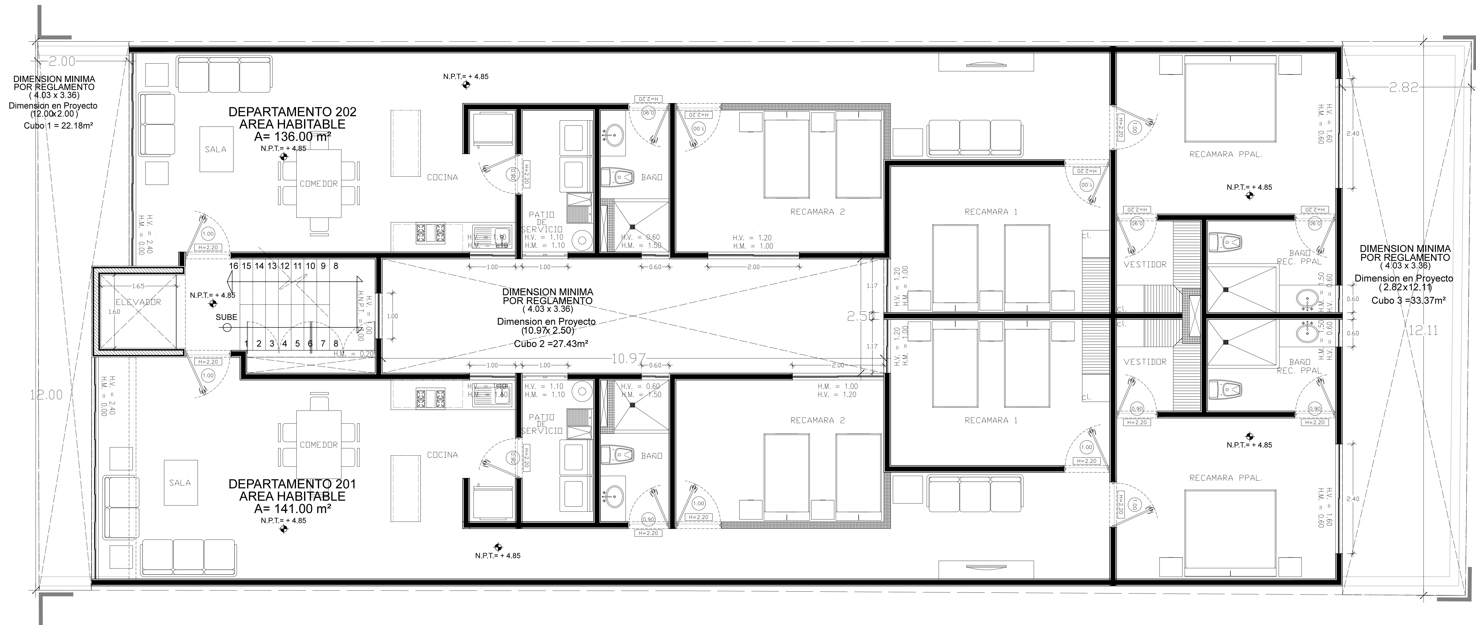
PLANTA TIPO AMORES 48
