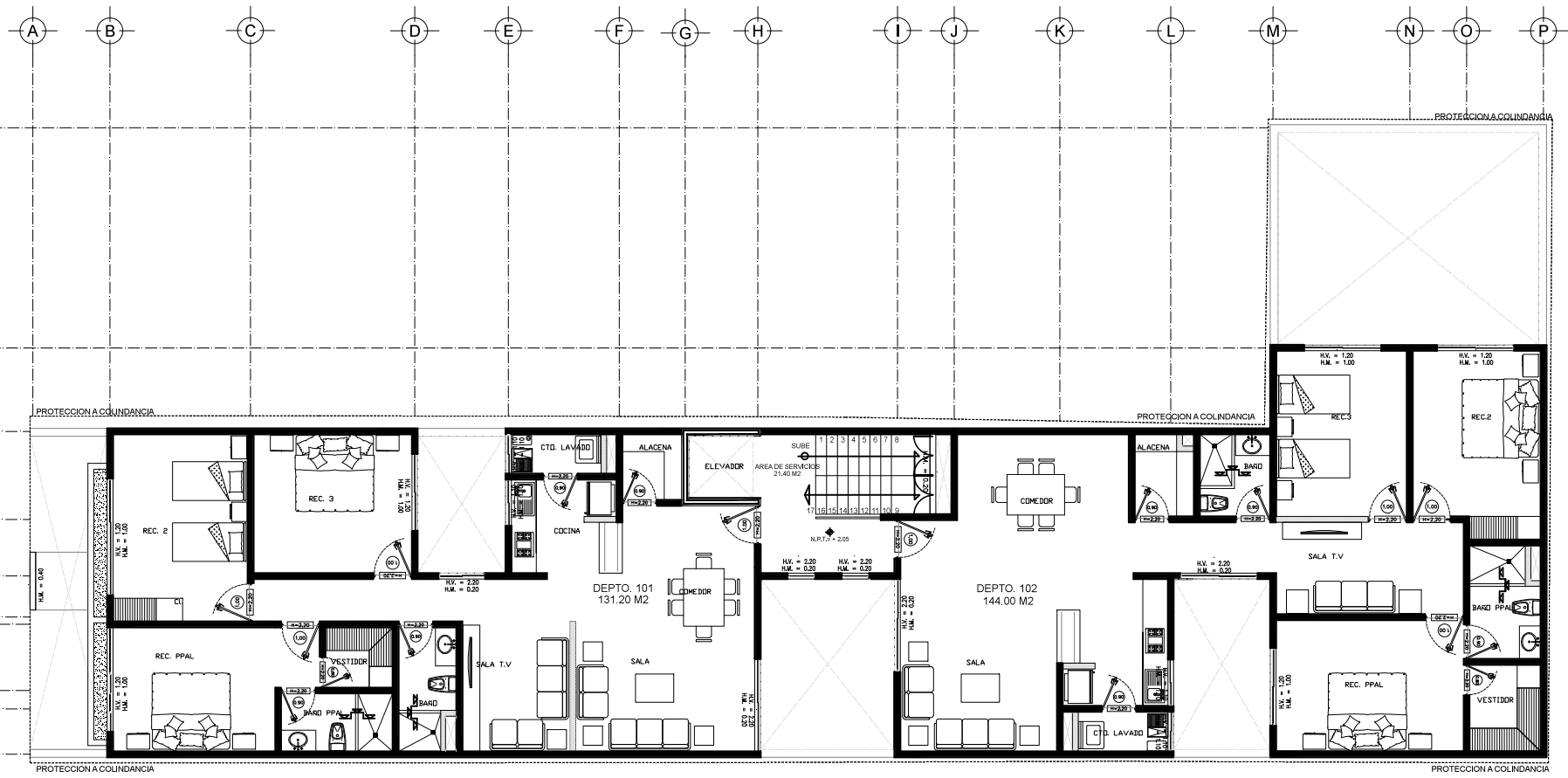
PLANTA PRIMER NIVEL NICOLAS SAN JUAN 838
